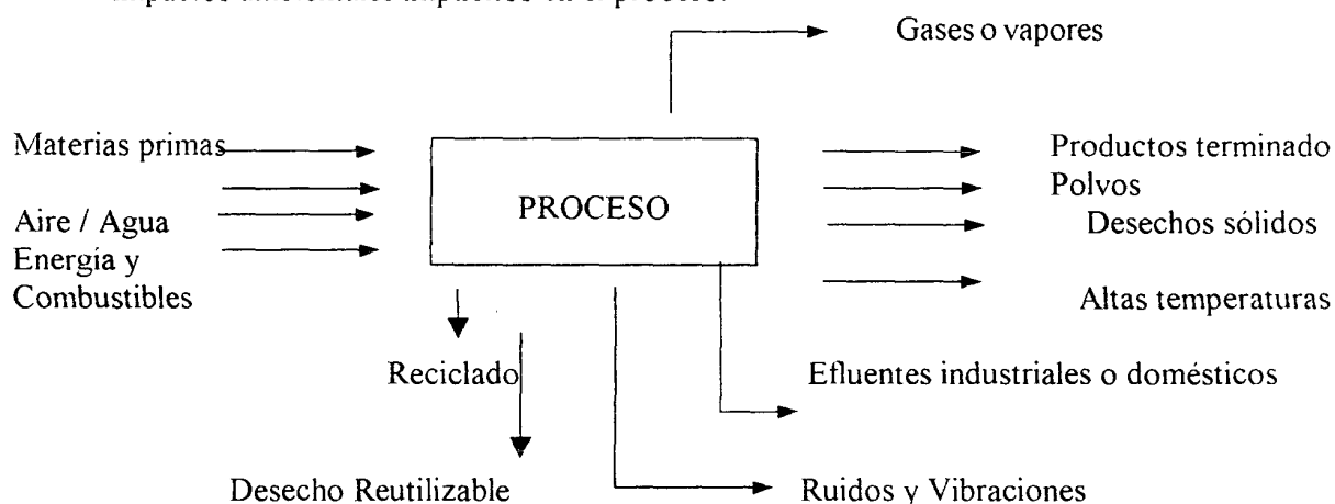
Figura 4.3 Componentes básicos de un balance de materiales
