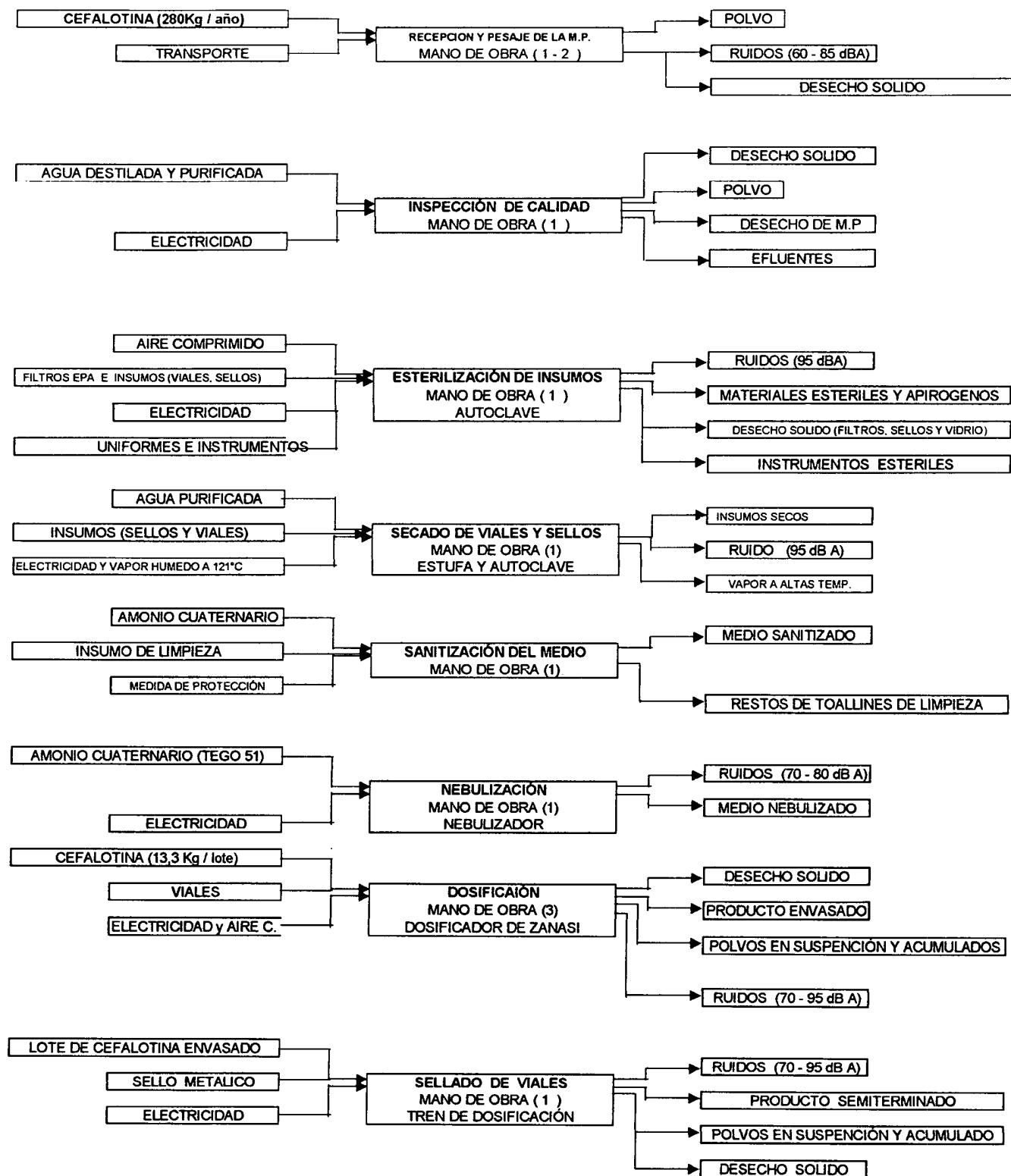
Figura 5.2 Diagrama de bloque para la producción de Cefalotina Inyectable
