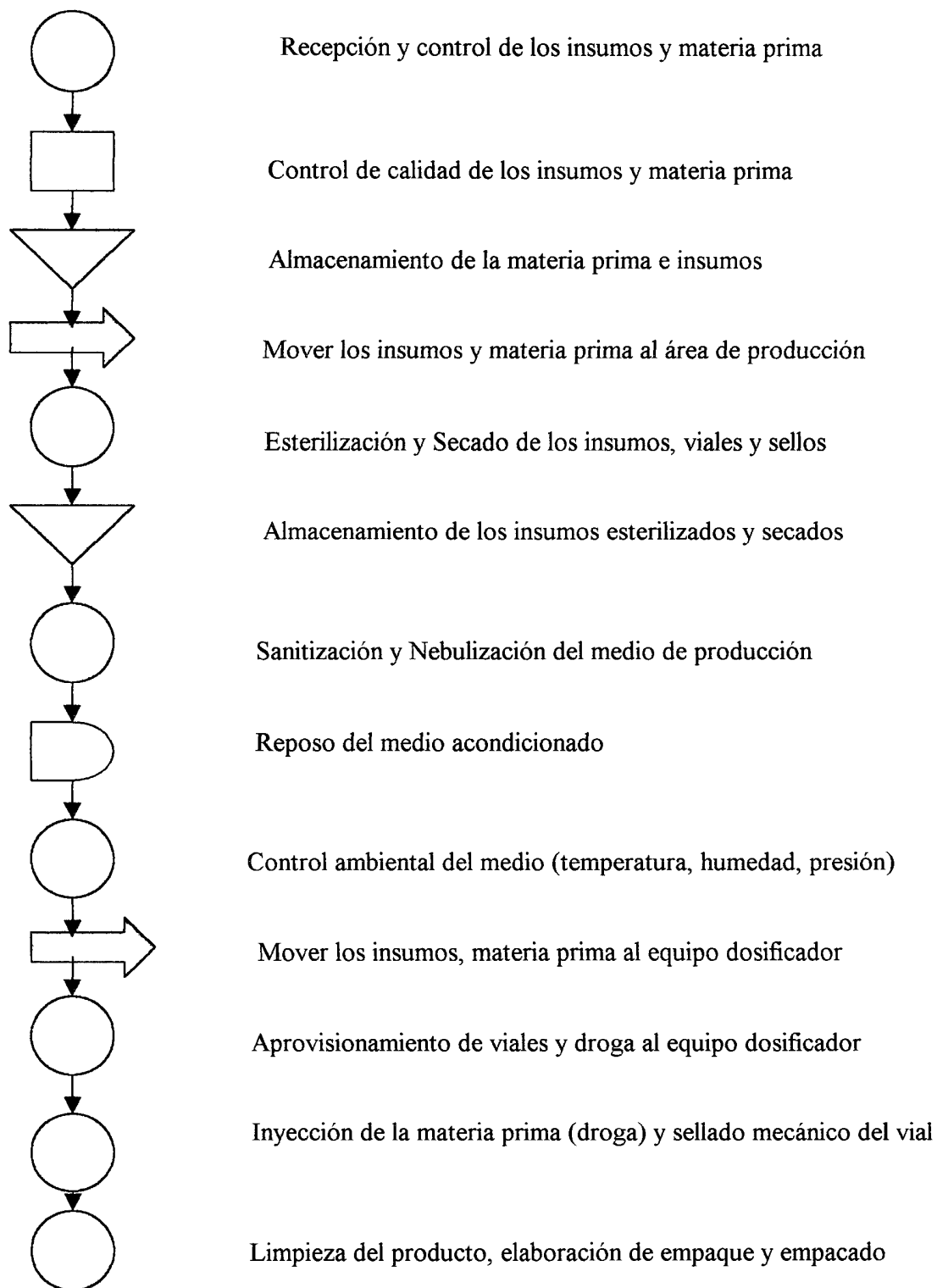
Figura 5.1 Resumen del Diagrama de Operación del Proceso
