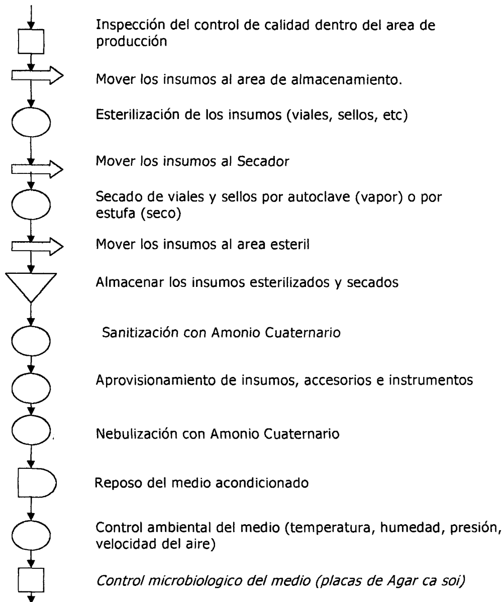
Figura H2. Continuación diagrama de operación de proceso Fuente: Rojas, 2005
